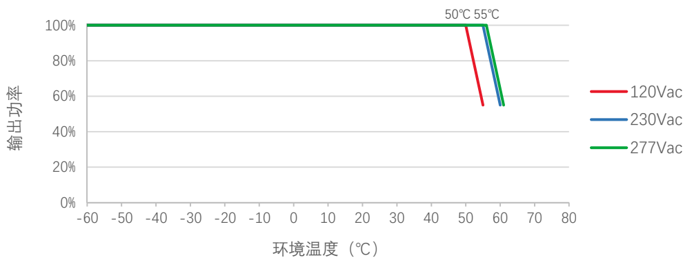
降额曲线
