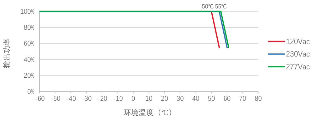
降额曲线
