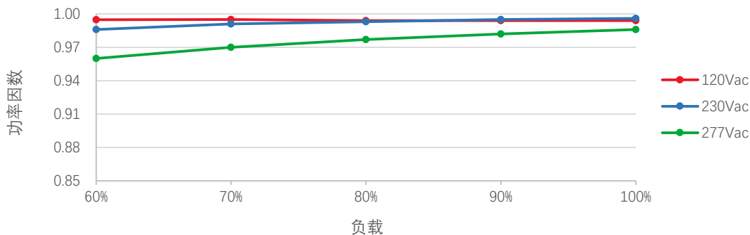
总谐波失真曲线
