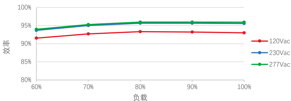
效率曲线 ( I_o=1.05A )
