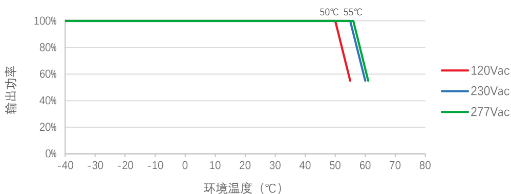
降额曲线
