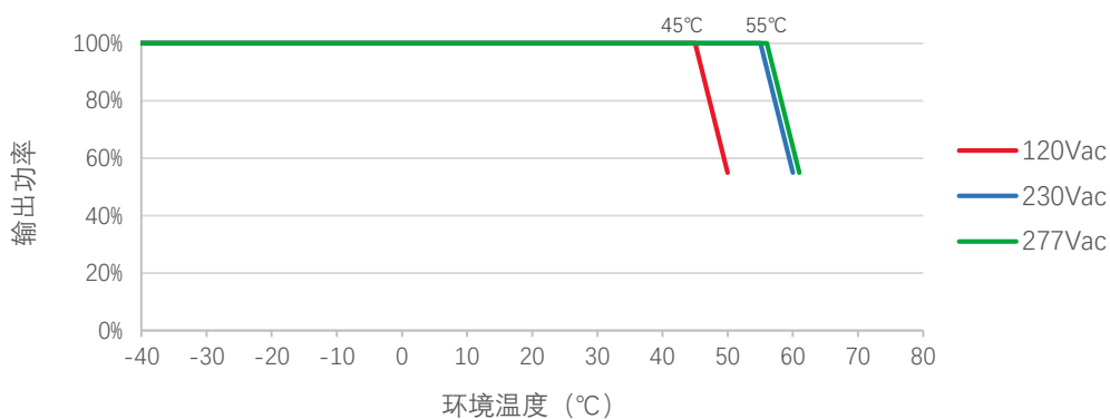
降额曲线
