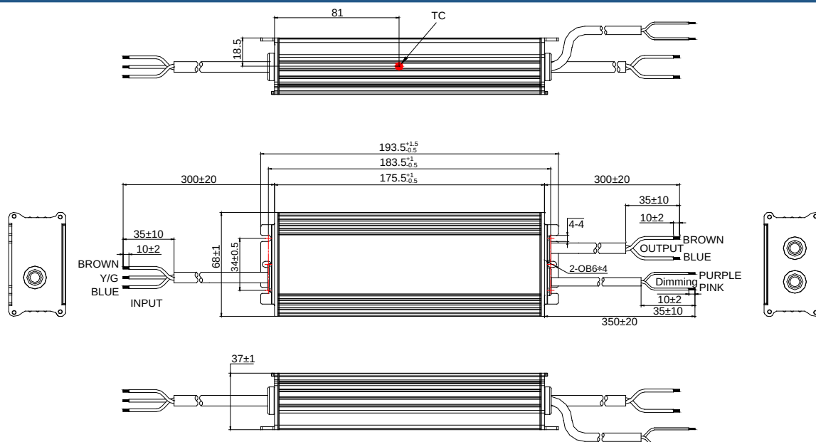
结构尺寸示意图
