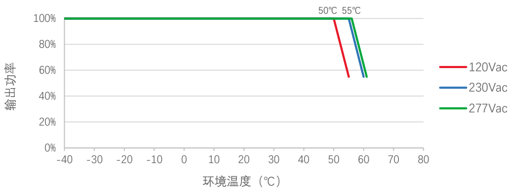
降额曲线
