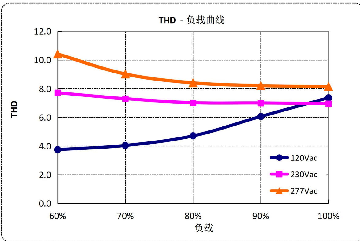
总谐波失真曲线
