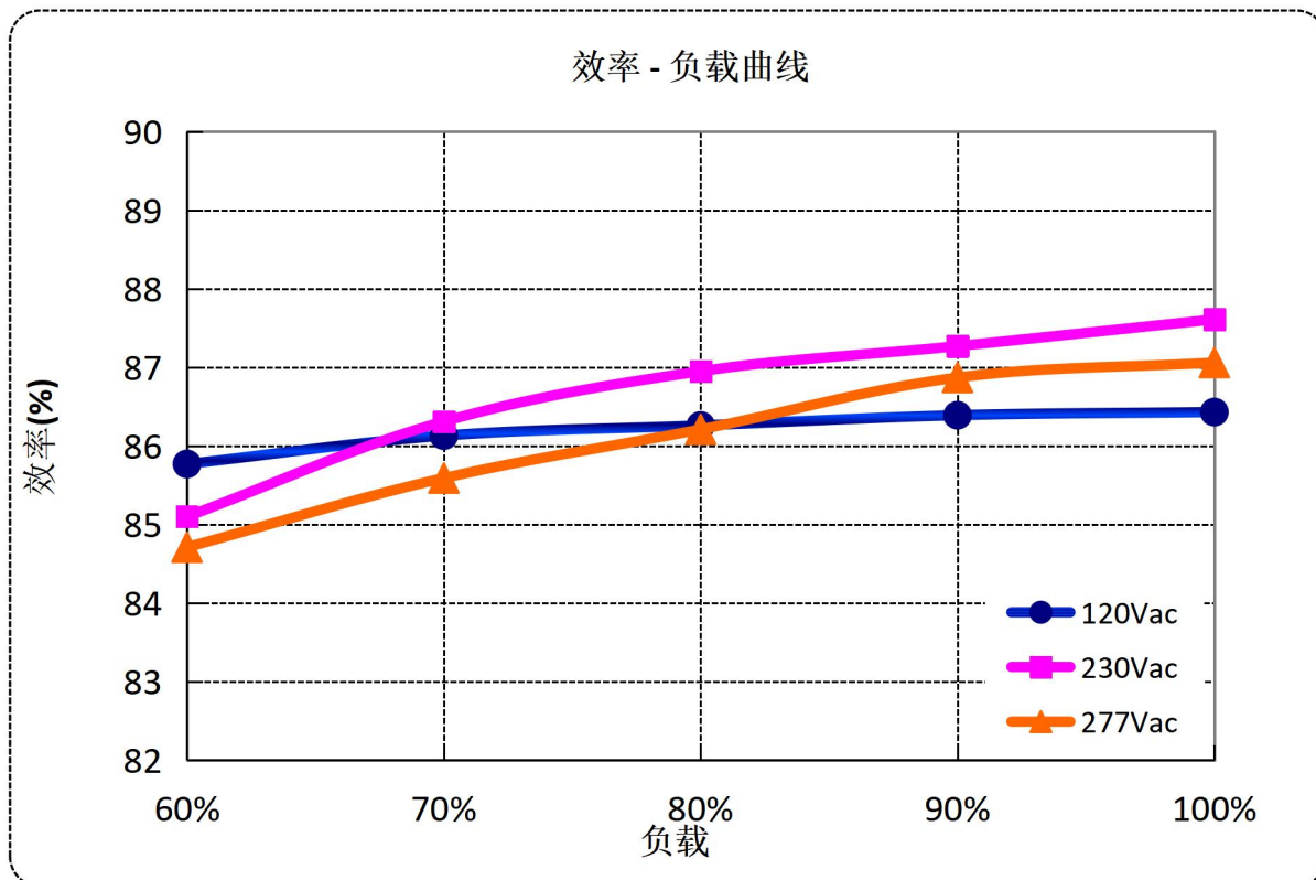
效率曲线
