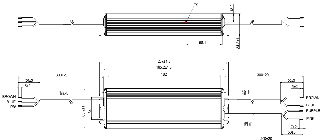
结构尺寸示意图
