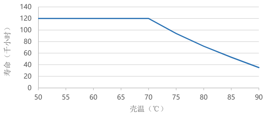
寿命曲线
