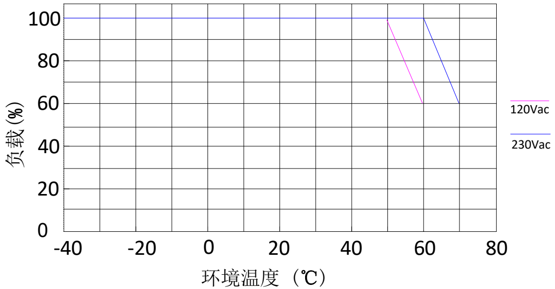
降额曲线
