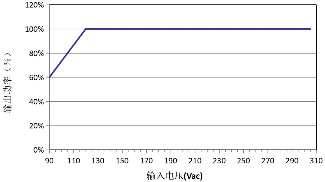
输出功率—输入电压曲线
