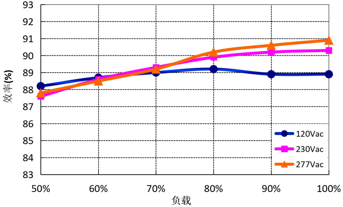
效率 - 负载曲线
