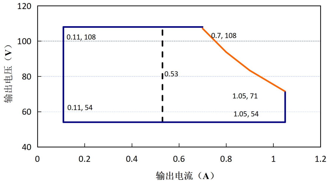
输出电压/输出电流曲线
