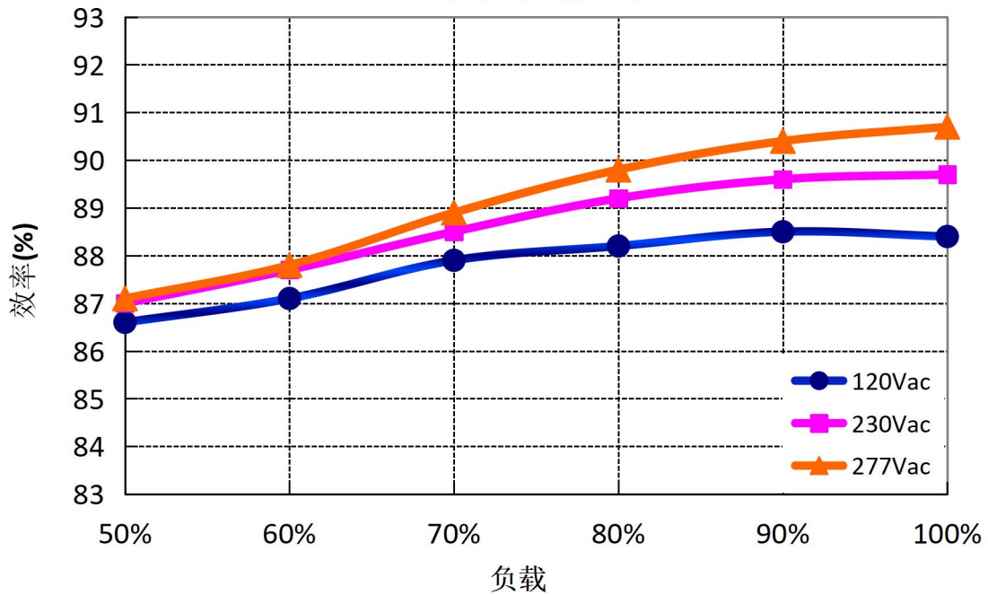
效率 - 负载曲线
