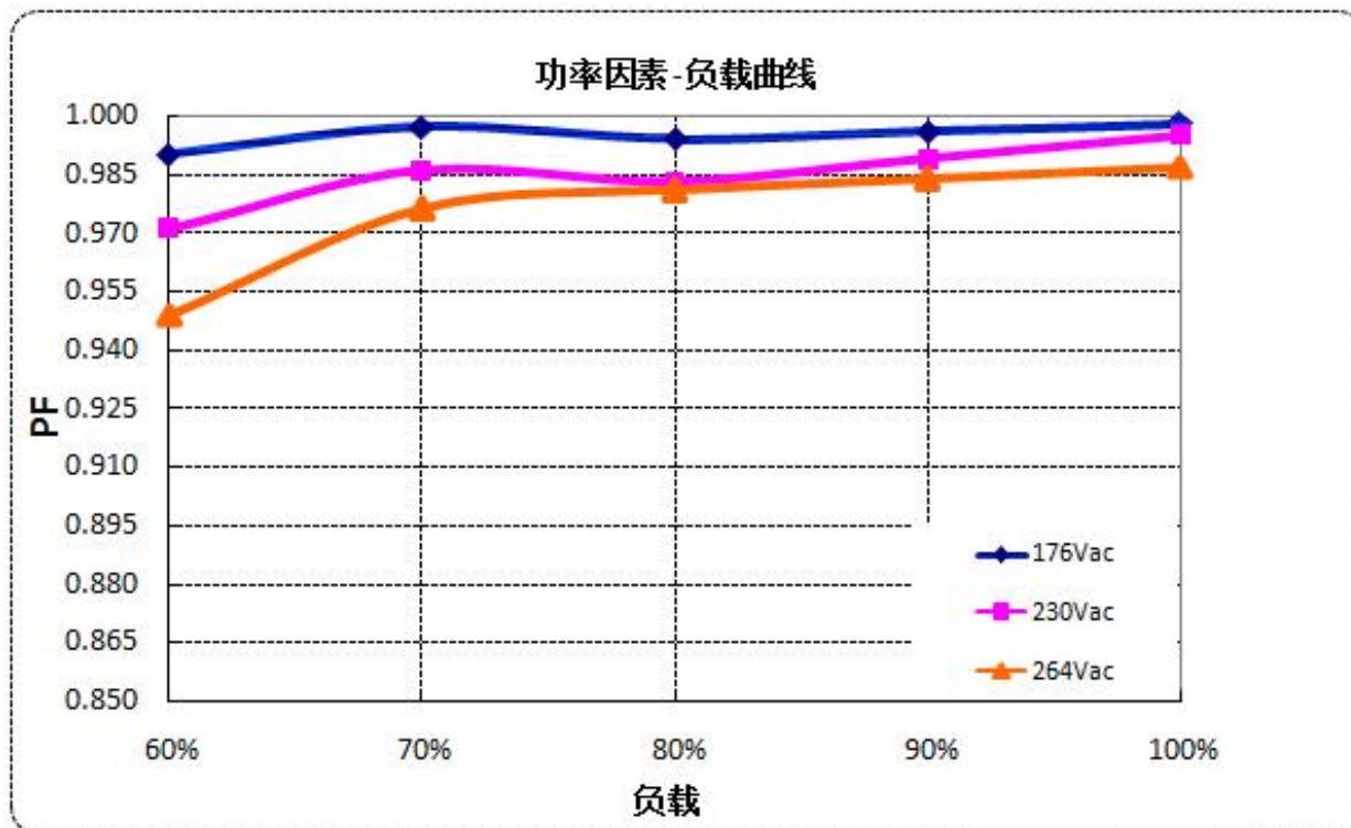
功率因数曲线
