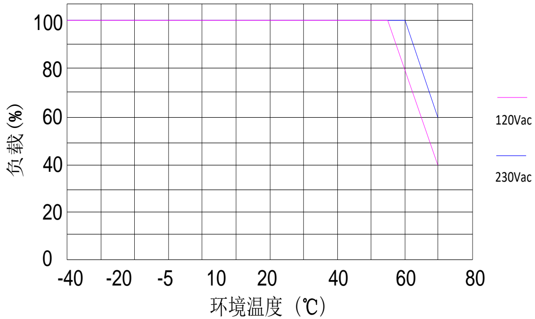
降额曲线
