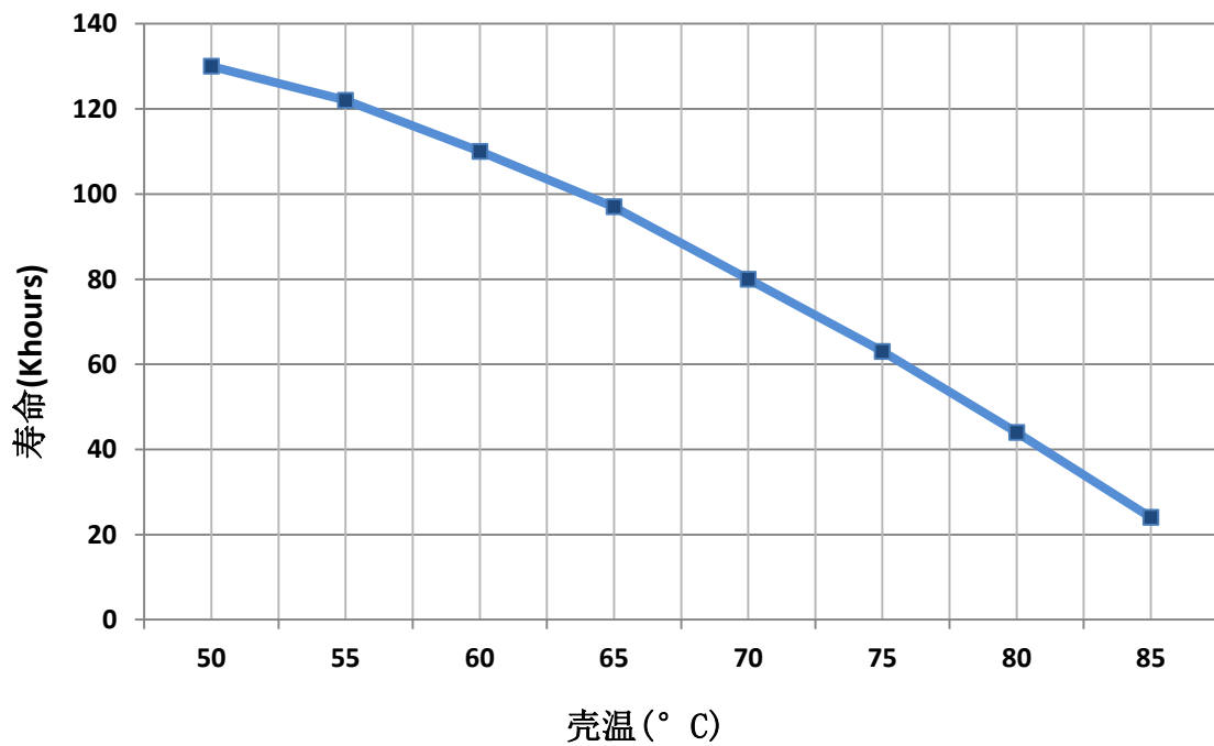
寿命 - 壳温曲线
